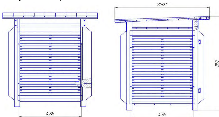
Рисунок 1 – Габаритный чертеж будки для самописцев БС-1
